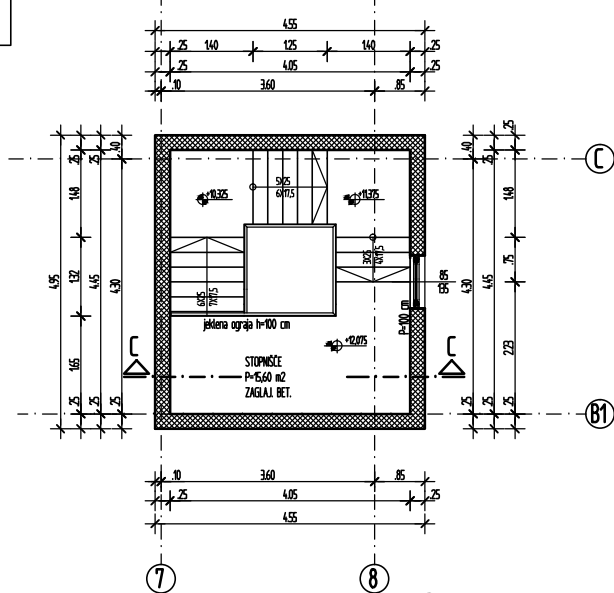
TLORIS ETAŽA +12,075 1:100
